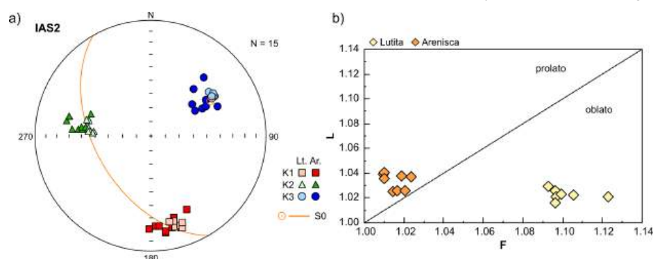
Figura 2. a) Proyección estereográfica de los ejes del elipsoide de la estación IAS2. k_1 , k_2 y k_3 representan los ejes máximo, intermedio y mínimo, respectivamente; lutitas (Lt.) y areniscas (Ar.). b) Diagrama de Flinn, donde se observa una distribución bimodal controlada por la litología.
